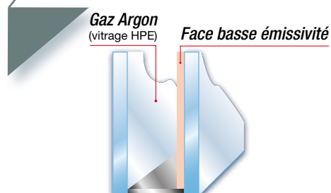
Double vitrage isolant 4/16/4 FE ou HPE avec ou sans Warm Edge (menuiseries en rénovation)
